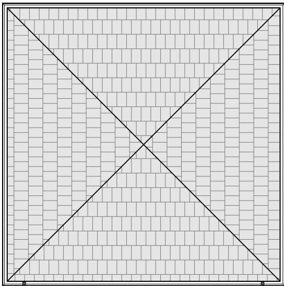
Roof Plan 1 : 100
